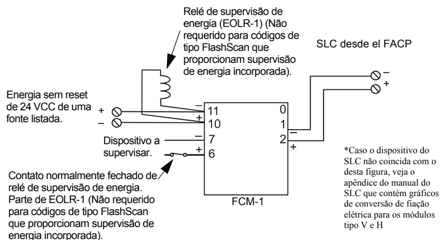
Figura 4.1 Ativação de supervisão de energia externa com utilização de relés
