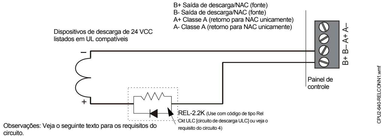
Figura 4.6 Conexão estilo típico 4 de um dispositivo de descarga ao painel de controle
