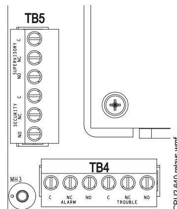
Figura 3.22 Conexões de relé de formato C
