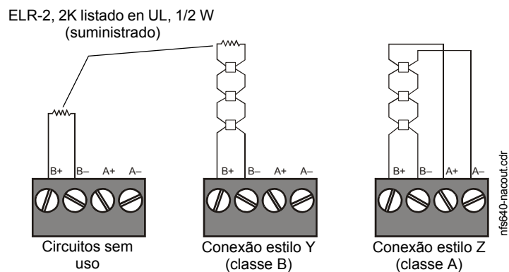
Figura 3.20 Conexões de Circuitos de aparelhos de notificação (NAC)
