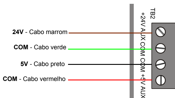
Figura 3.19 Conexão com a saída de acessório do TB2 em CPS-24/E
