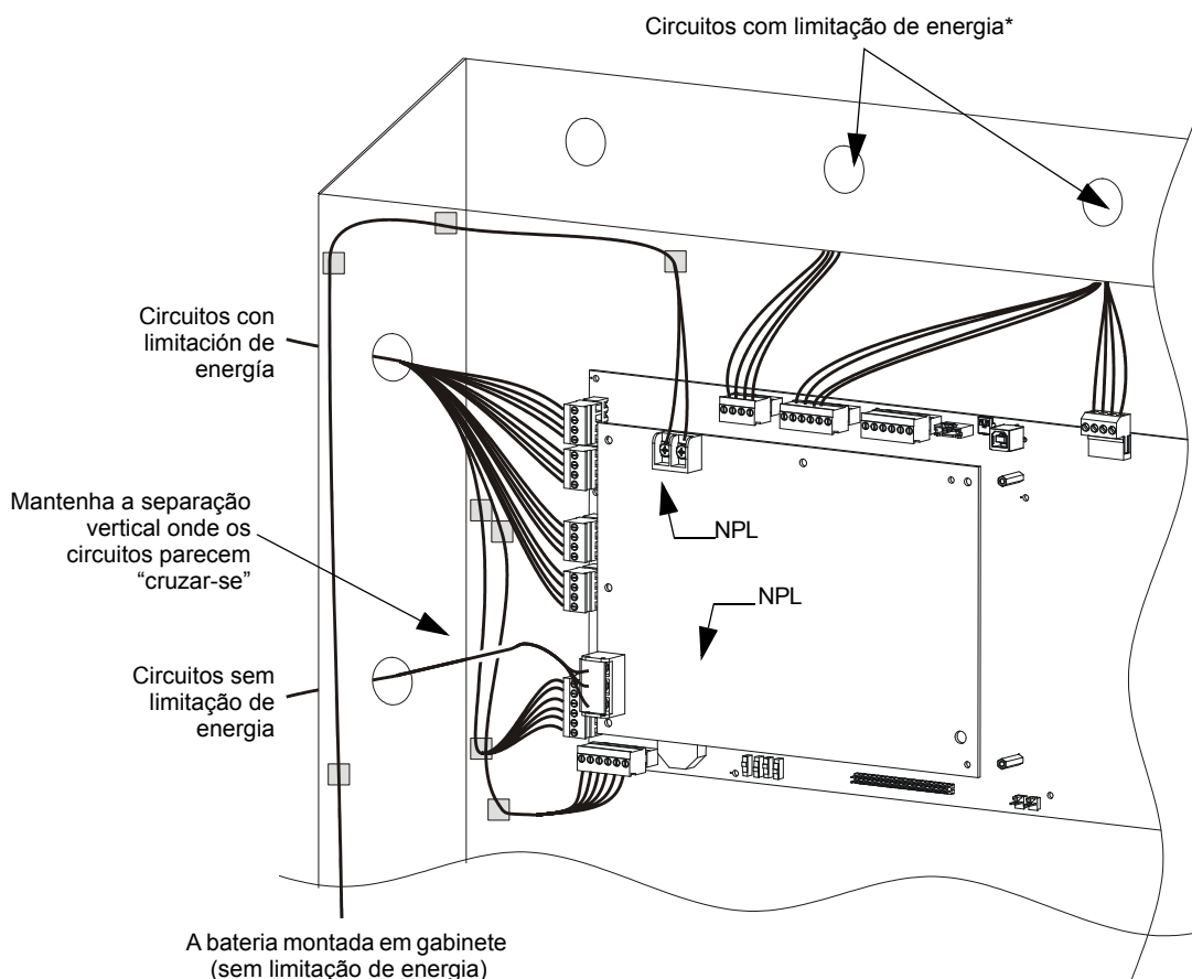
Figura 3.24 Requisitos típicos de UL para fiação elétrica com limitação de energia (Mostra-se com os relés conectados com módulos com limitação de energia)
