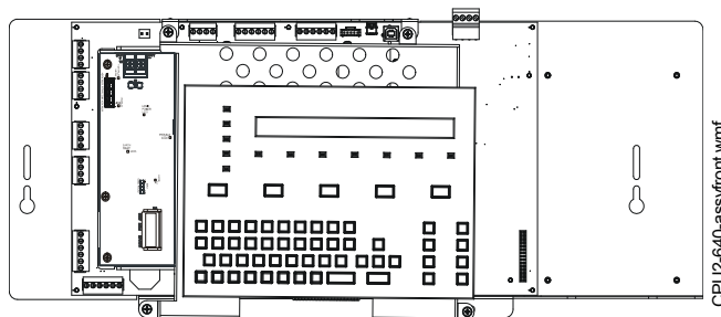
Figura 2.1 Painel de controle NFS2-640/E com unidade de teclado/tela opcional instalada
