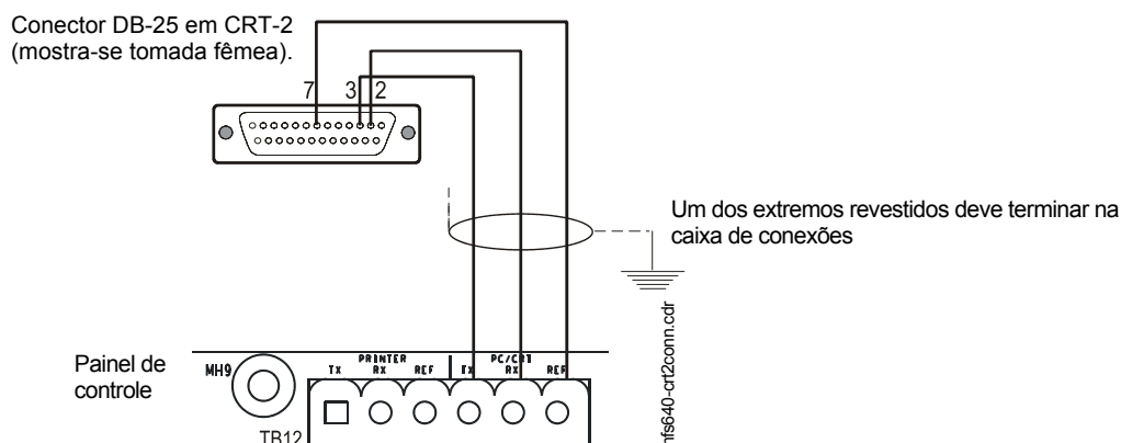
Figura 3.28 Conexão de um CRT-2
